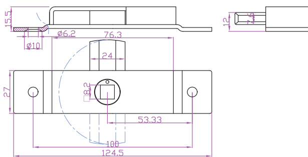
锁体
