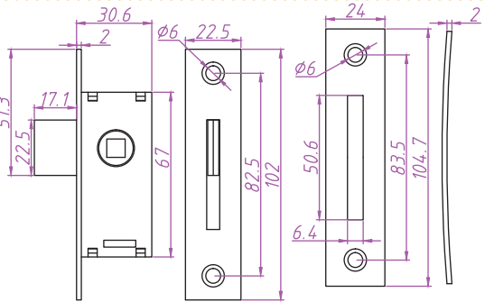
锁体
